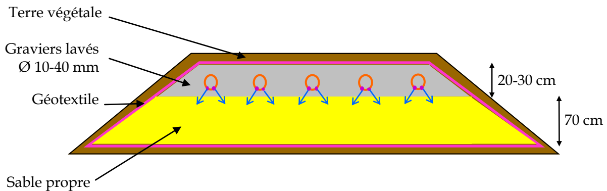
Coupe transversale
