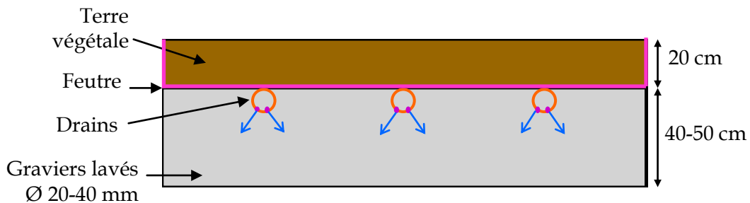
Coupe transversale
