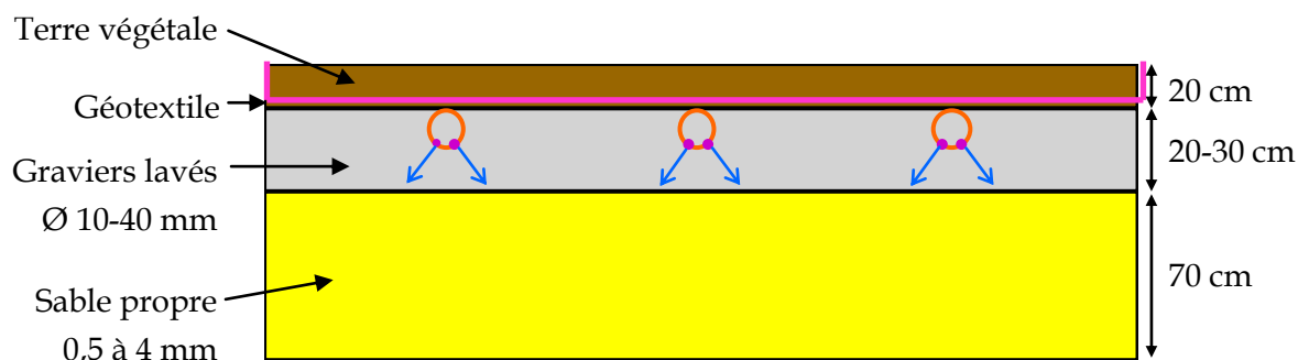
Coupe transversale
