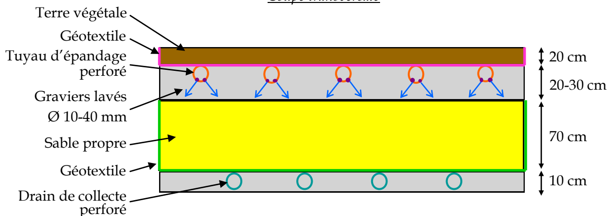
Coupe transversale
